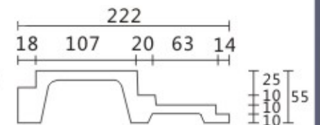
BG-8066 2400×222×55
