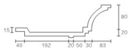
BG3001-415
