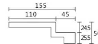
BG-6075 2400×155×50
