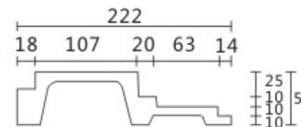
BG-8066 2400×222×55
