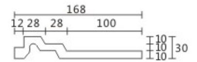
BG-6068 2400×168×30
